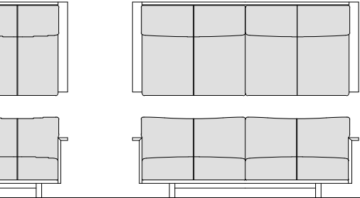
Sofa 189 W189. D87.5. H75. SH38
