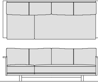
C Sofa 221 W221. D87.5. H75. SH38
